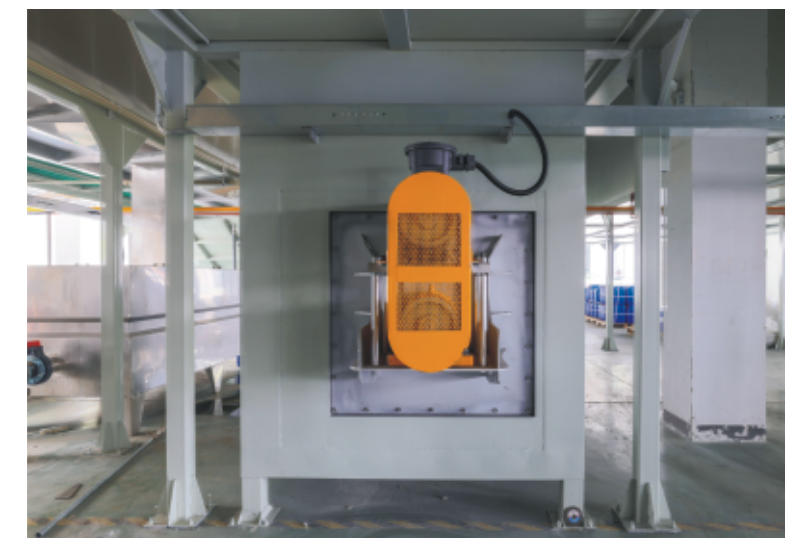
插入式循环风机 Plug in circulating fan
